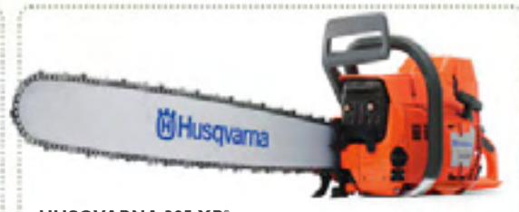
HUSQVARNA 395 XP® 93,6 см³, 4,9 кВт, длина шины 45–90 см, 7,9 кг. Air Injection™ и Low Vib. Имеется модификация с подогреваемыми рукоятками и карбюратором. Поставляется в Россию.
